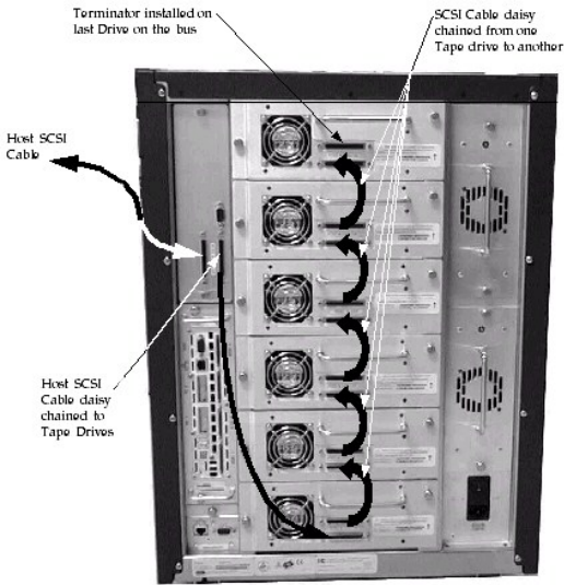
그림 8. 호스트에서 SCSI 케이블 연결
