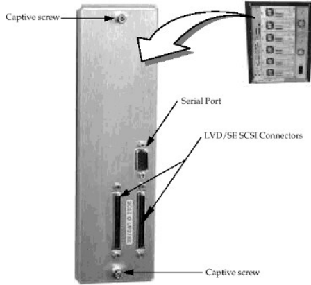
그림 5. Host SCSI 인터페이스 PCBA
