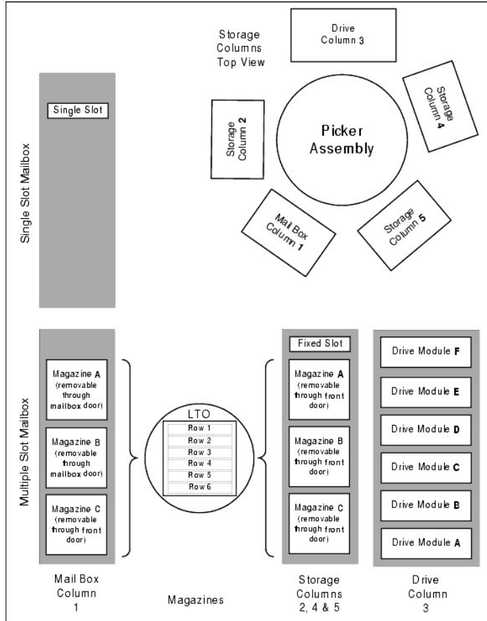
그림 6. 스토리지 칼럼 지형도
