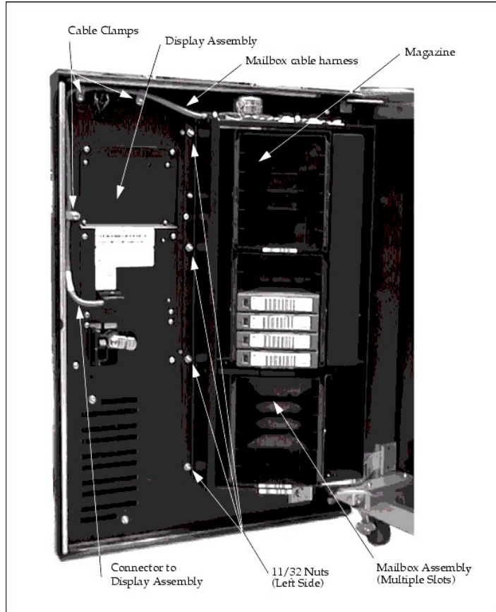
그림 5. 다중 슬롯 메일박스 설치하기
