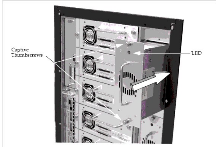
그림 3. 중복형 DC 전원 공급장치 설치하기
