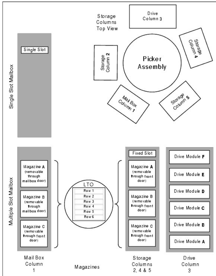
그림 3. 스토리지 컬럼 구성요소와 좌표 시스템
