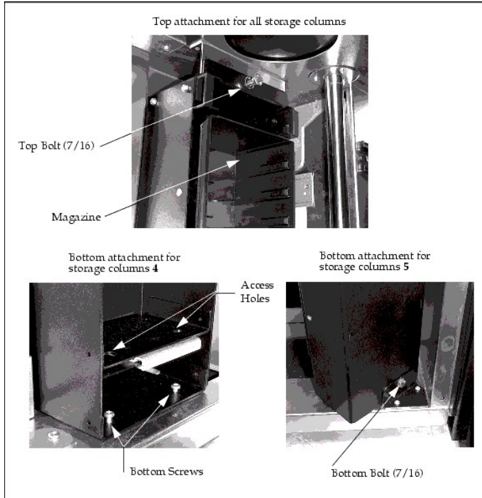
그림 7. 스토리지 칼럼 설치하기
