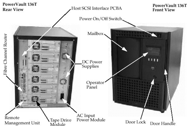
그림 1. Dell PowerVault 136T LTO 라이브러리
