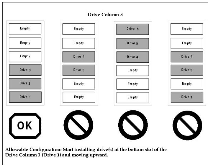
그림 1. 테이프 드라이브 모듈 가용 구성도
