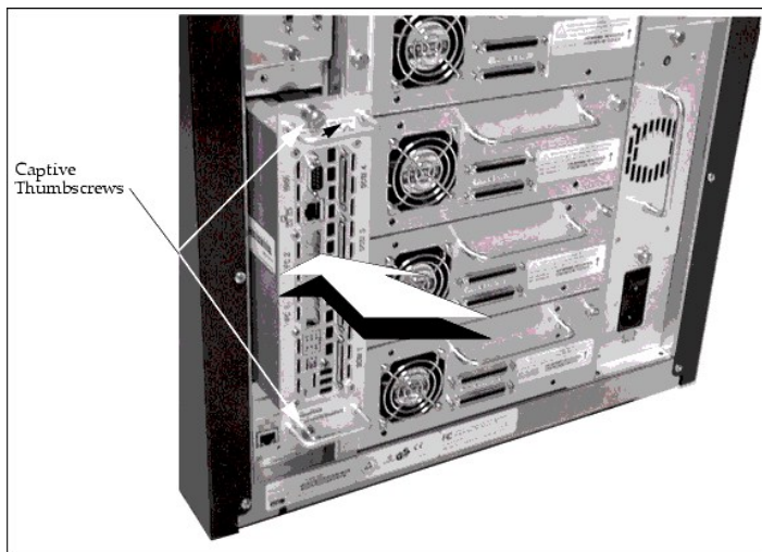
그림 4. Dell PowerVault 136T 파이버 브리지 설치하기
