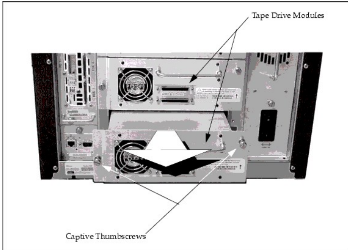
그림 2. 테이프 드라이브 모듈 설치하기
