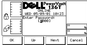
그림 80. 셋업 > 유틸리티 > 보안 > 비밀번호 입력 대화상자
