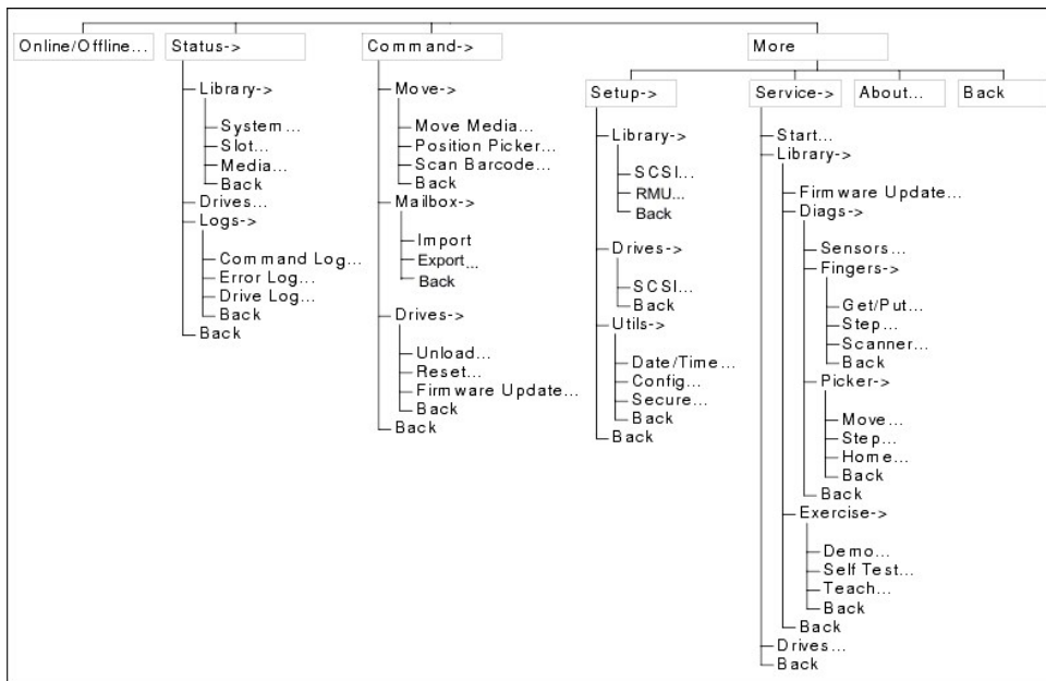
그림 1. 메뉴 트리
