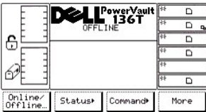
그림 17. 오프라인 대화상자
